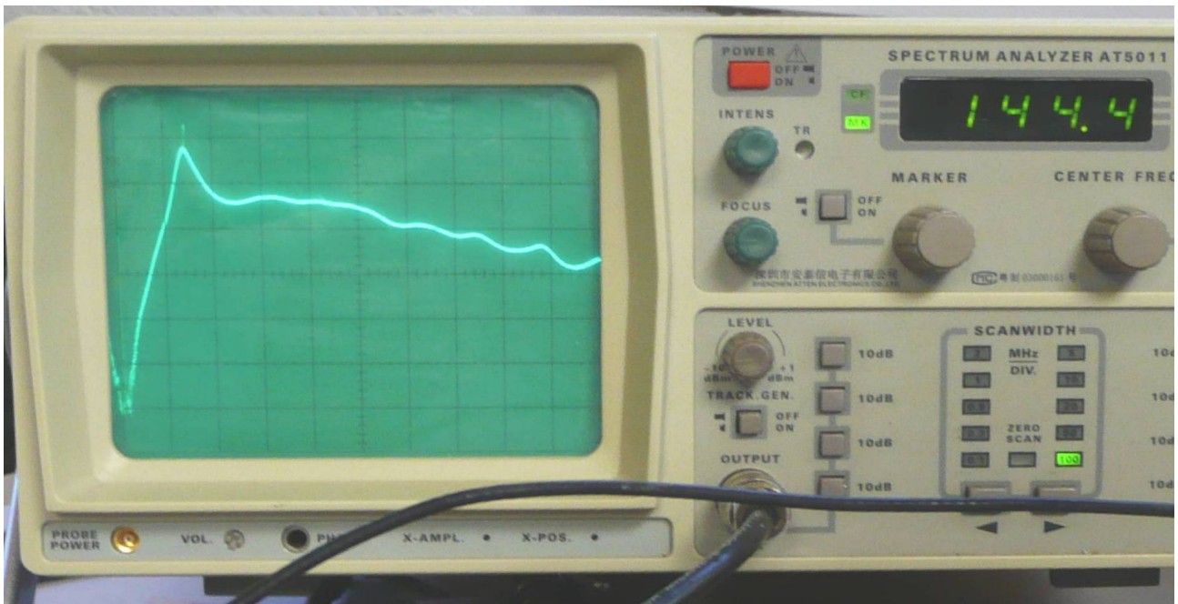
CURVA DE RESPUESTA 0-1GHz sin filtro
