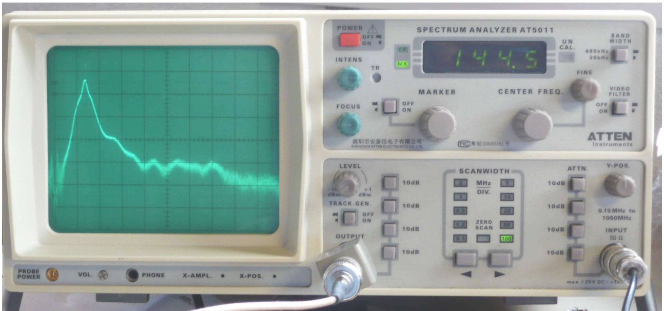
CURVA DE RESPUESTA 0-1GHz con filtro
