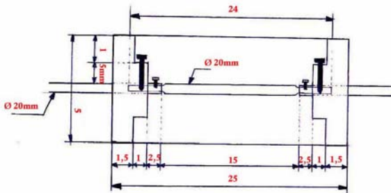
Detalle de la bobina
