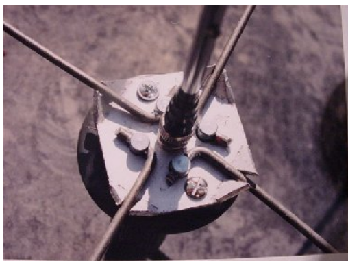
a) Detalle base \frac{1}{4} onda de mano
