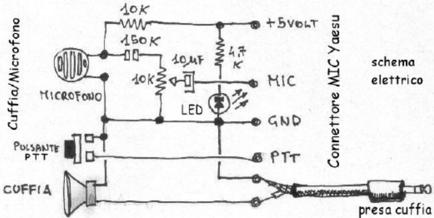
adattatore Cuffia/Microfono per computer – rtx YAESU FT-897-857-817
